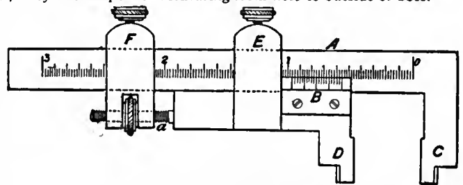
FIG. 70.—Vernier Caliper.
