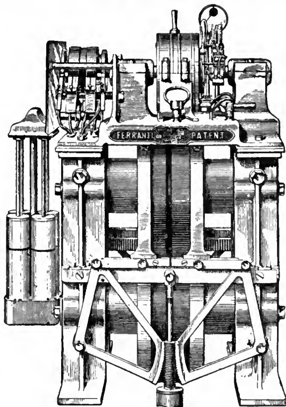
FIG. 11.—Ferranti Rectifier.
