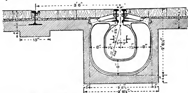
FIG. 6.—Section of Side Conduit.
