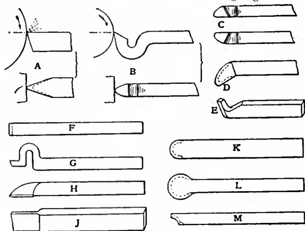
FIG. 2.—Metal-turning Tools.
