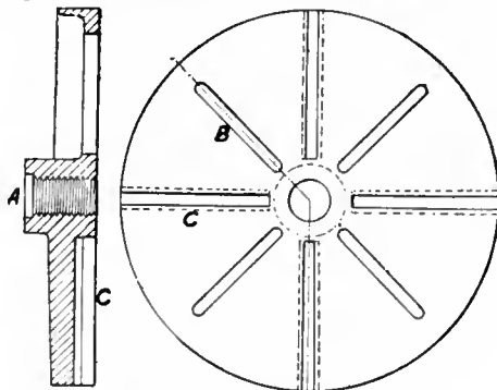
FIG. 37.—Face-plate.
